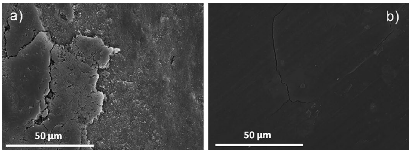
Figura 7. Micrografía de MEB de las superficies desgastadas de los composites nSiC/CNFs: a) 80/20 y b) 20/80 %vol. sinterizados a 1600 °C/1 min.
