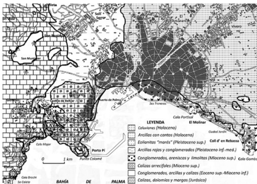
Figura 1. Esquema geológico de los alrededores de Bellver; simplificado de OLMO ZAMORA, P. del, M. ÁLVARO LÓPEZ y J. RAMÍREZ DEL POZO. Mapa geológico de España, escala 1:50 000, hoja 698/723 (iv), Palma . Madrid: IGME, 1991.
