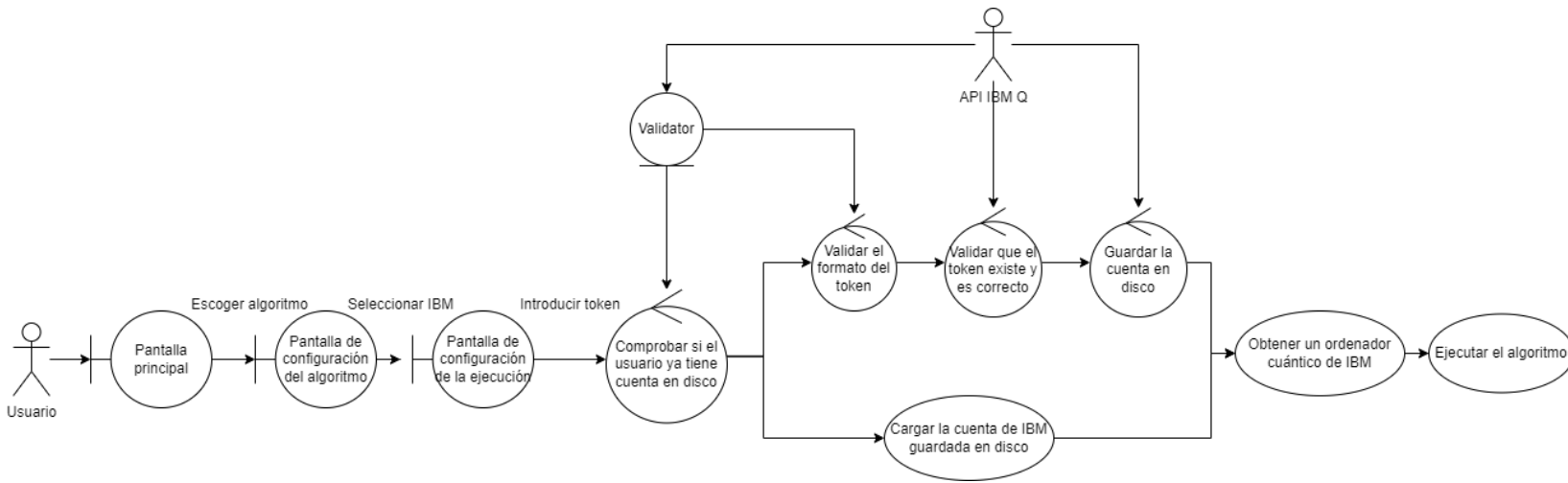
Figura 7.4: Diagrama de robustez - Activar cuenta de IBM
