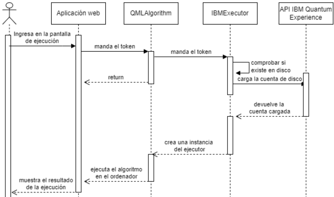
Figura 8.3: Diagrama de interacción - Cargar la cuenta de IBM guardada en disco
