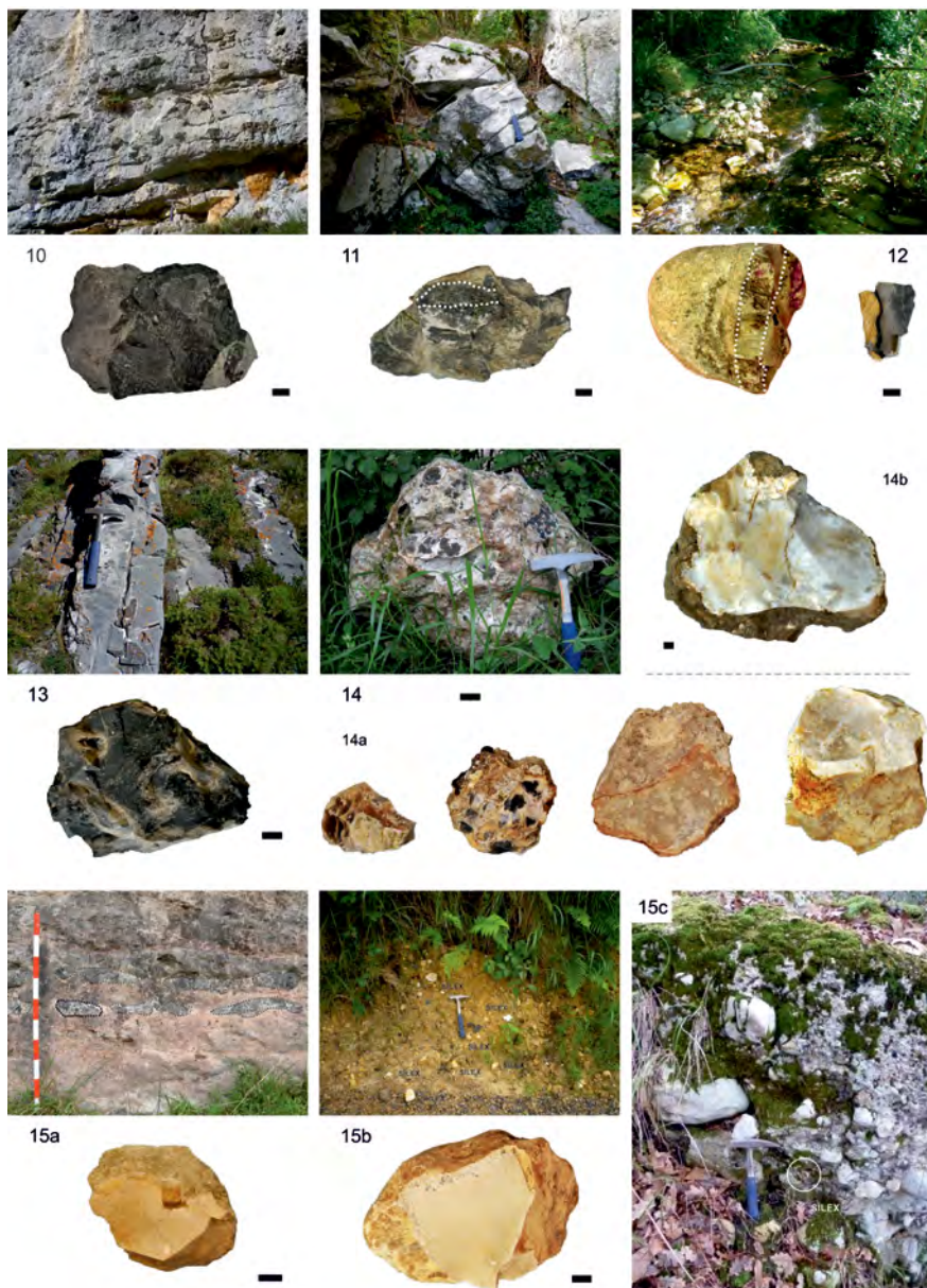
Lám. 2.—Ejemplos de sílex geológicos: 10, Caliza de Peña Redonda. Cantera de Pelúgano (Aller); 11, Paquete Tendeyón. Congostinas (Lena); 12, Aluvión en el río Mampodre, a la altura de Bada-Tospe (Parres); 13, Fm. Escalada. Pico de la Capilla (San Isidro, Aller); 14, Sílex de Piedramuelle, bloque en un muro —hoy desaparecido— en una casa del El Picural (Piedramuelle, Oviedo); 14a, Sílex de Piedramuelle, bloques recogidos en superficie en el área de Piedramuelle (Oviedo); 14b, Sílex de Piedramuelle recogido en Los Barredos (Oviedo); 15, Sílex de Piloña; 15a, El Pandotu (Piloña); 15b, Alteritas en Los Rebollinos (Coya, Piloña); 15c, Conglomerado de Miyares (Piloña). Salvo indicación todas las muestras están recogidas en el corte o zona próxima. Escala: 1 cm. Martillo geológico: 28 cm. Fotos E. Duarte.
