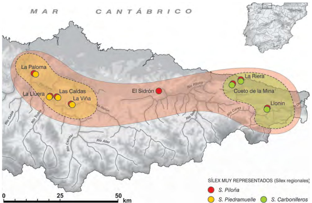
Fig. 4.—Principales áreas de distribución espacial de los sílex asturianos muy representados. En rojo: sílex de Piloña; en amarillo: sílex de Piedramuelle; en verde: sílex carboníferos.
