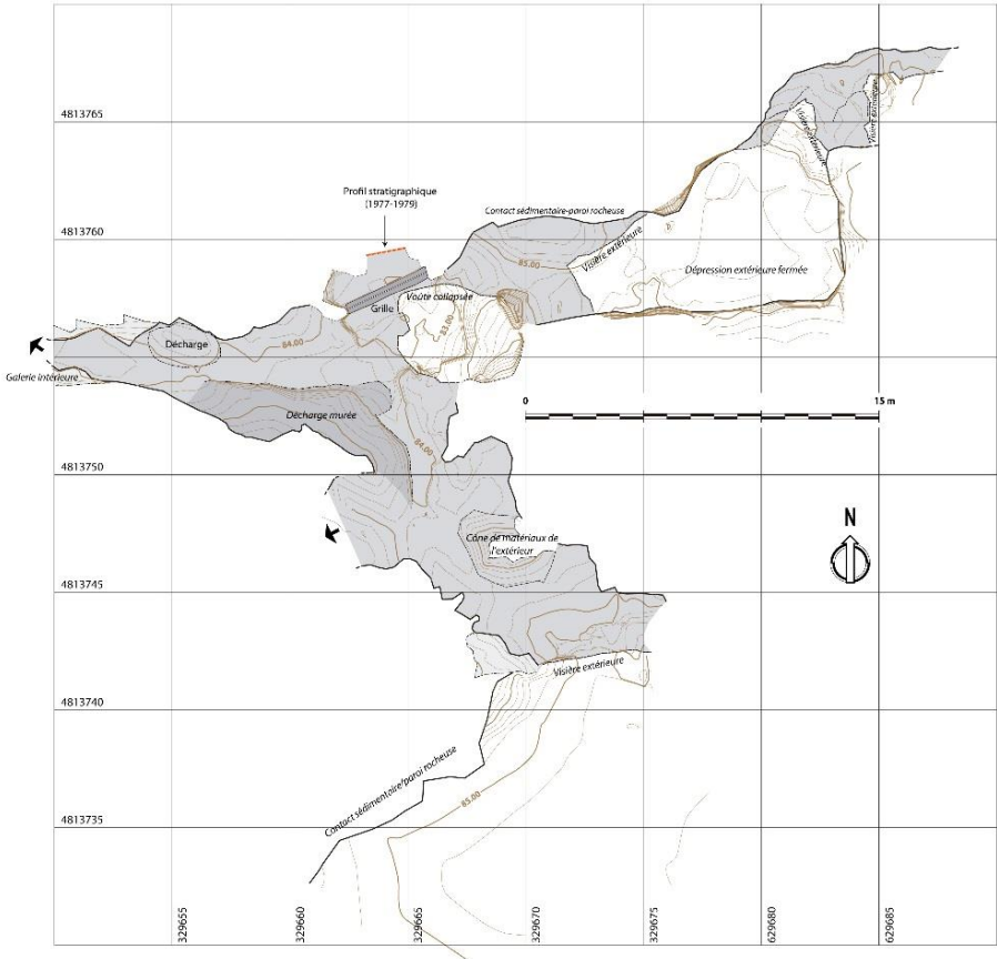
Figura 2. Plano topográfico de la cueva de El Cierro (realización Luis Teira).
