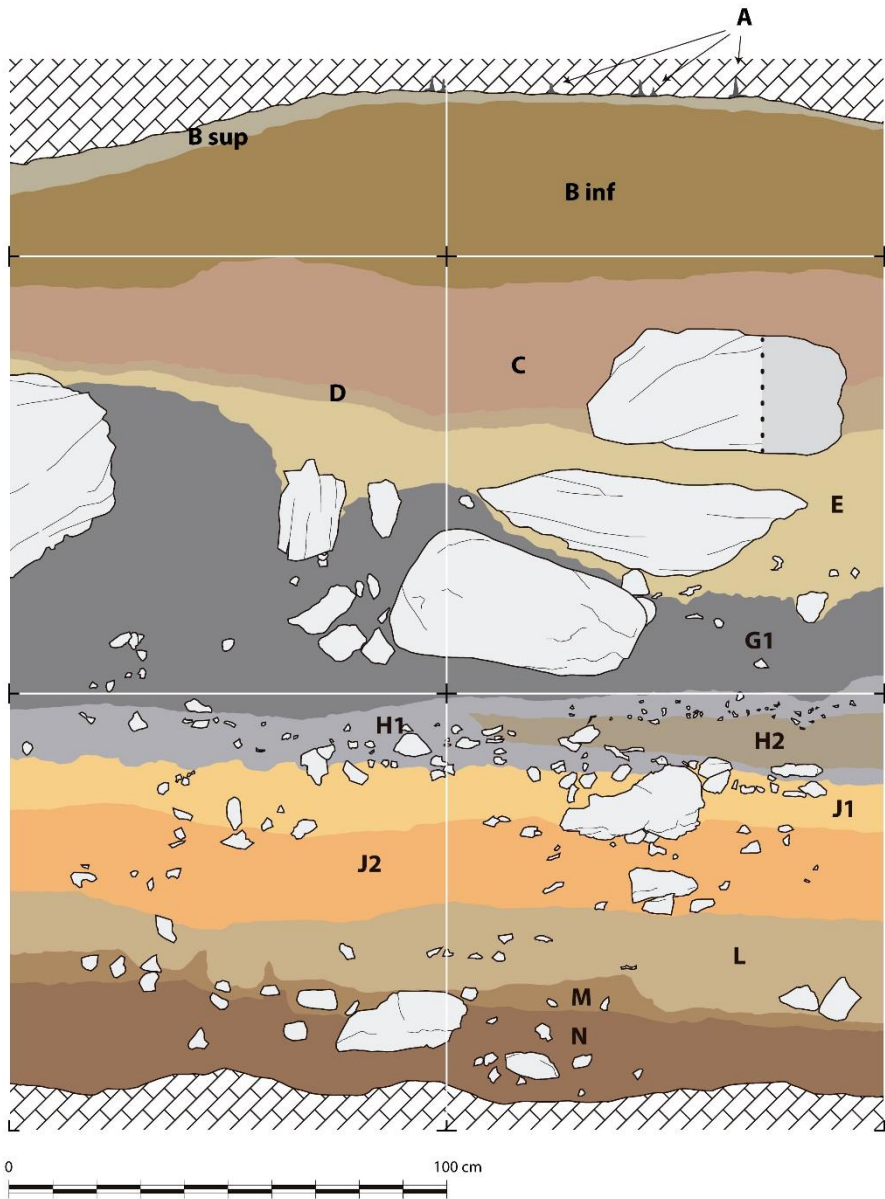
Figura 3. Sección estratigráfica del yacimiento de la cueva de El Cierro después de la limpieza realizada en la campaña de 2014 (realización Luis Teira).
