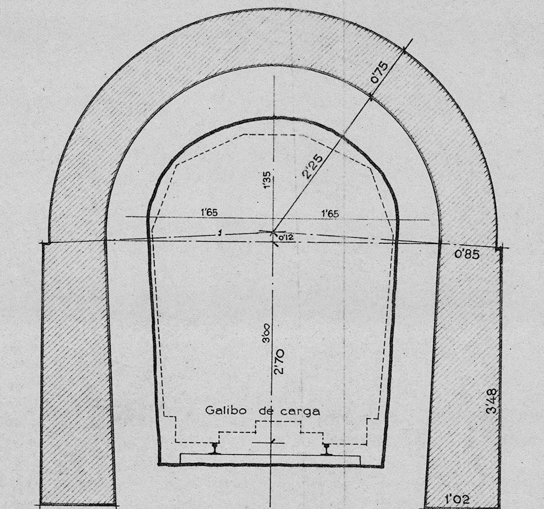
Secciones mínima y de reconstrucción Escala 1:50
