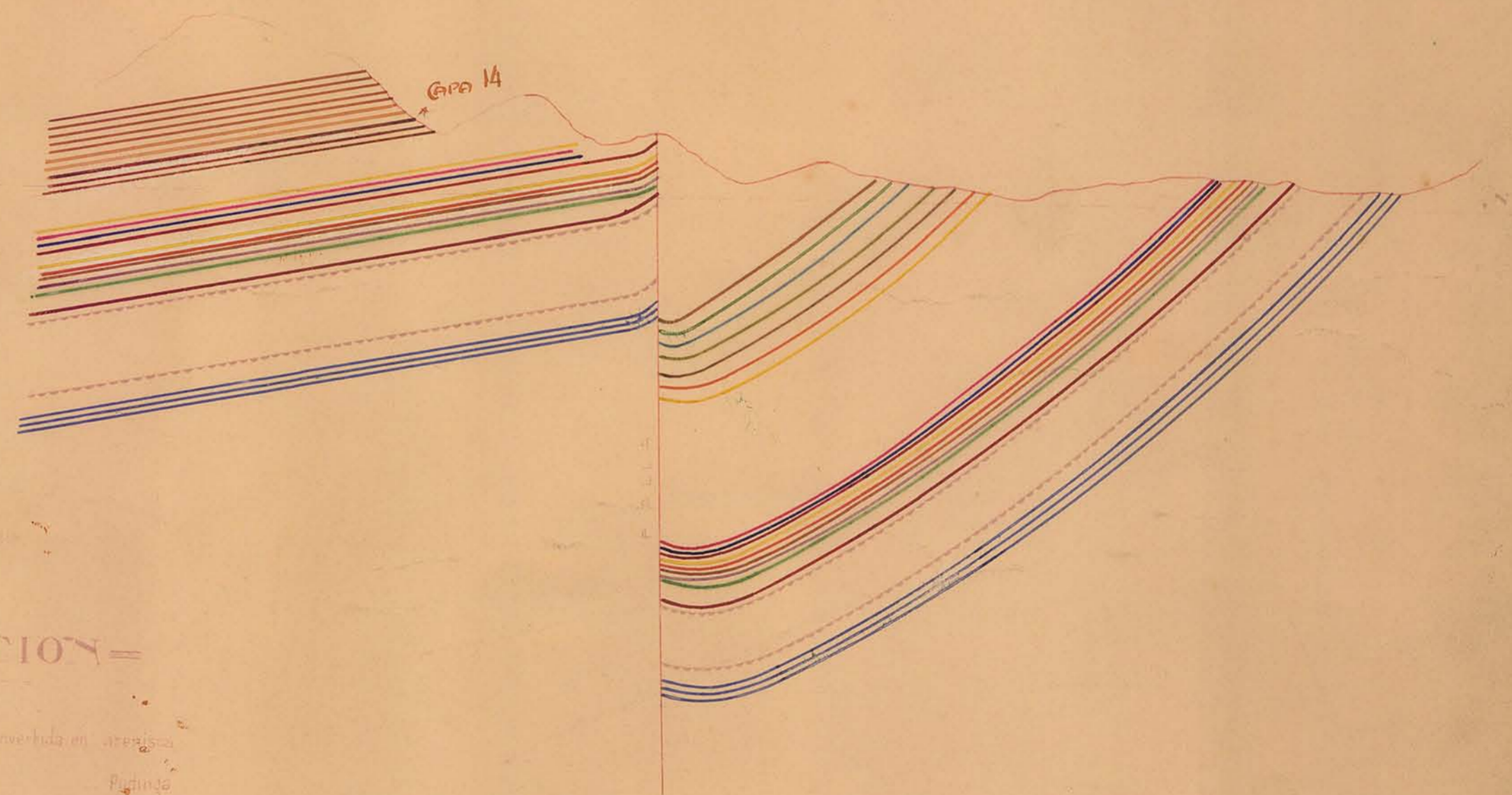
CORTE POR H-I-J-K
