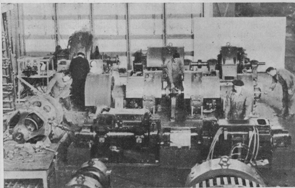
Totalidad de la maquinaria del equipo propulsor del buque "Artabro" en pruebas de taller, fabricados por la Constructora Nacional de Maquinaria Eléctrica de Reinosa.
