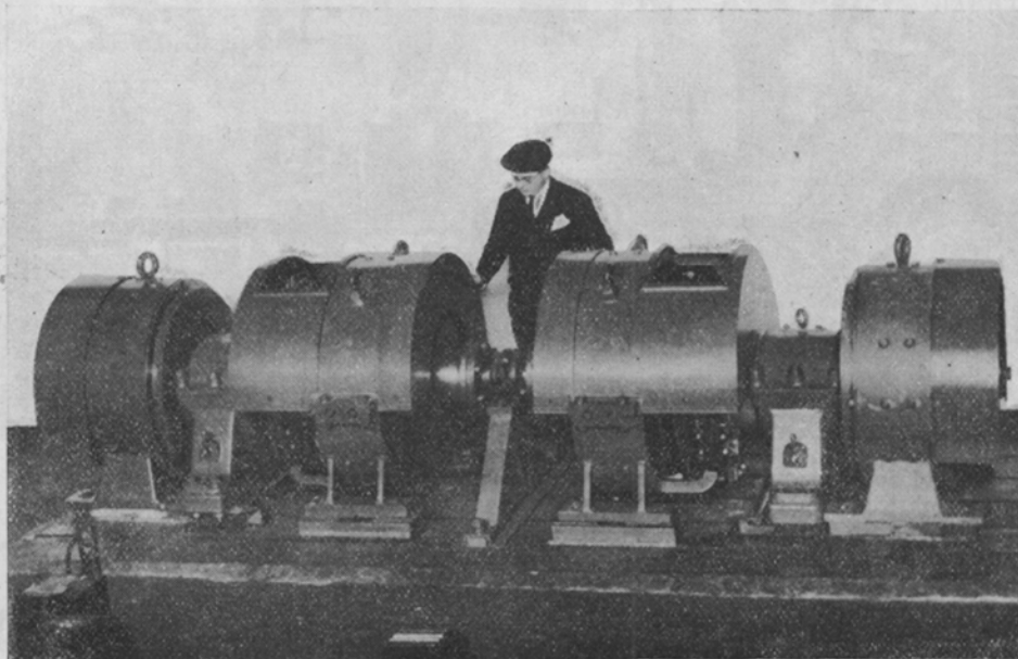
Dos generadores de 205 Kws. con 2 excitatrices de 50 Kws. del equipo propulsor eléctrico del buque "Artabro", fabricados por la Constructora Nacional de Maquinaria Eléctrica de Reinosa.
