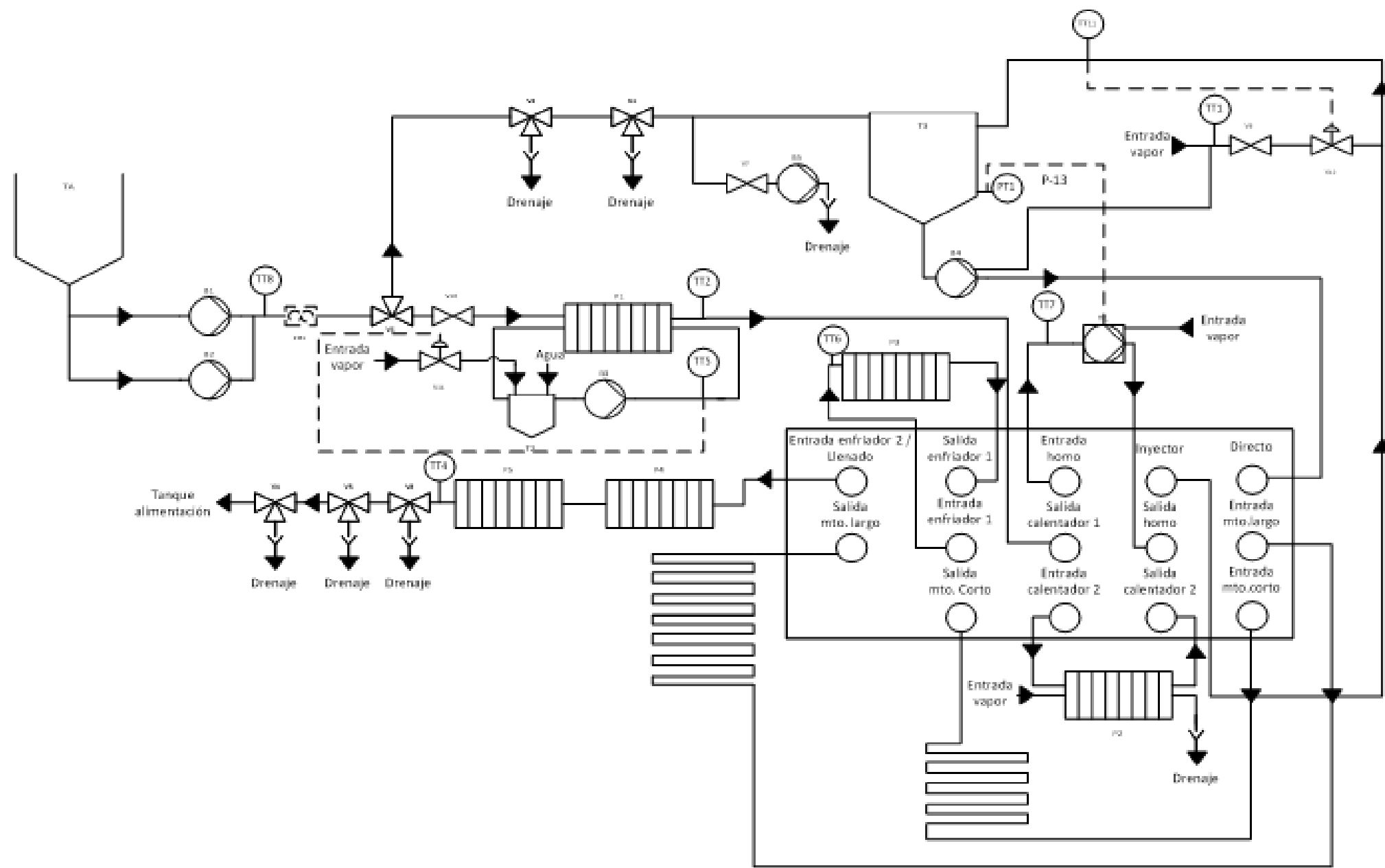
Esquema de proceso
