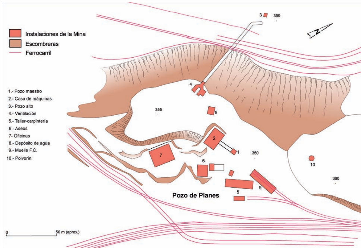
FIG. 5. Plano de las instalaciones mineras del pozo de Planes y su entorno, 1930. Cartoteca de la Fundación Río Tinto. Adaptado del original.
