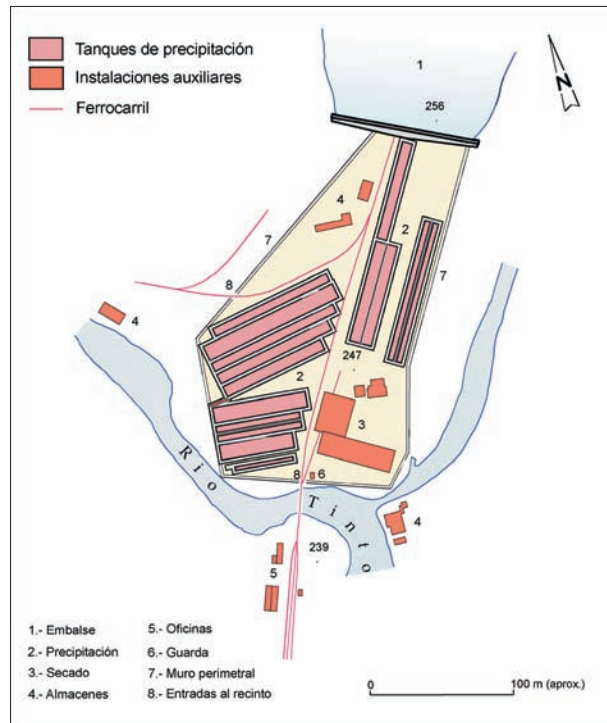
FIG. 7. Plano de las instalaciones de Cementación Naya, 1904. Cartoteca de la Fundación Río Tinto. Adaptado del original.
