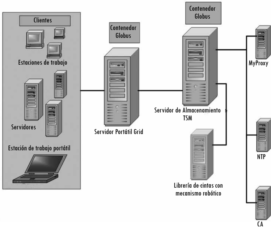
Figura 3. Arquitectura del prototipo para el sistema de almacenamiento masivo en el Cead
