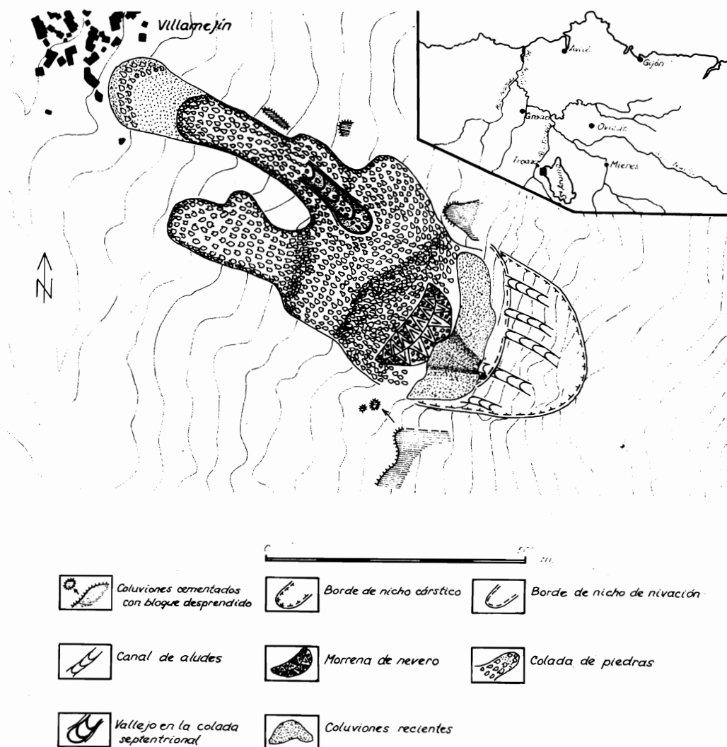
Fig. 4. Situación del área estudiada y croquis geomorfológico.
