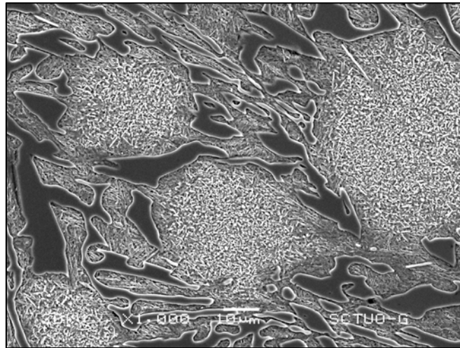
Figura 6.37 Fundición blanca alta en cromo con tratamiento de temple a 1050 °C y revenido a 525°C (1.000x)
