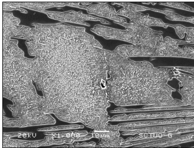
Figura 6.34 Fundición blanca alta en cromo con tratamiento de temple a 1000 °C y revenido a 500°C (1.000x)
