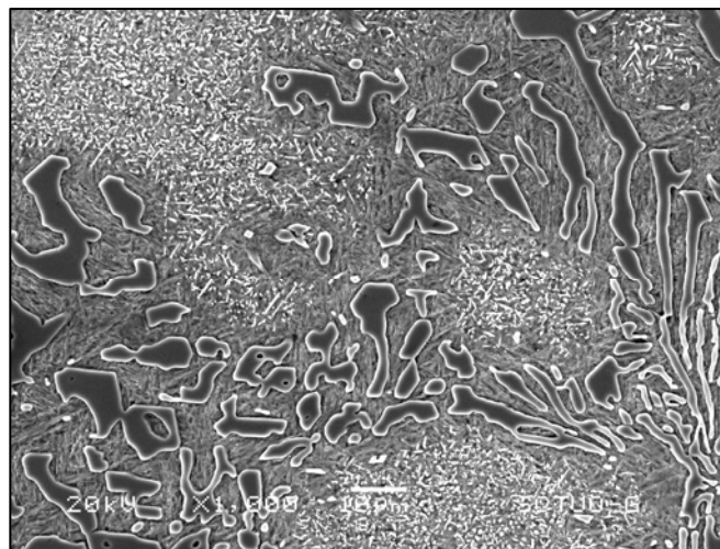
Figura 6.45 Fundición blanca alta en cromo con tratamiento de temple a 1050 °C y doble revenido a 525 °C (1.000x)
