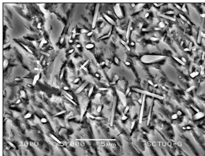
Figura 6.31 Fundición blanca alta en cromo con tratamiento de temple a 1.100 °C (5.000x)
