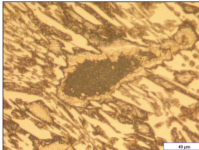
Figura 6.14 Fundición blanca alta en cromo con tratamiento de doble revenido a 500 °C (500x)
