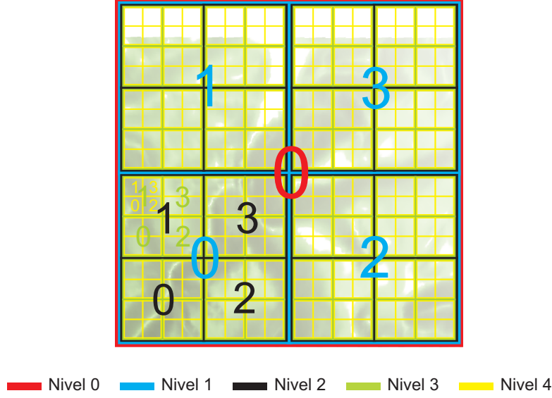
Figura 5.2: División estructurada de la geometría (II). Quadtree .
