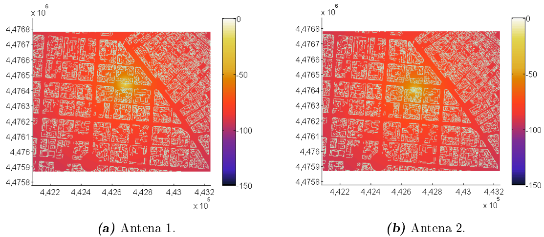
Figura 5.29: Ejemplo en entorno urbano (VII). Densidad de potencia total normalizada con el método empírico de Okumura-Hata, [dB].
