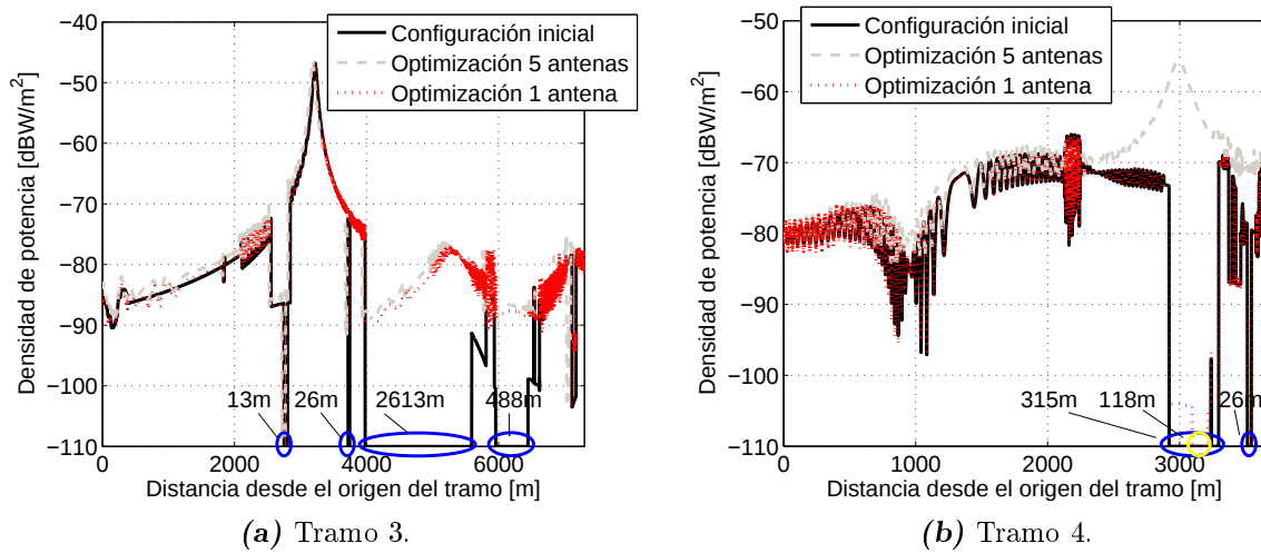
Figura 5.21: Ejemplo en entorno rural (VII). Densidad de potencia para la red GPRS a lo largo de un tramo del recorrido del convoy. Comparación entre la optimización con cinco estaciones y con una única.
