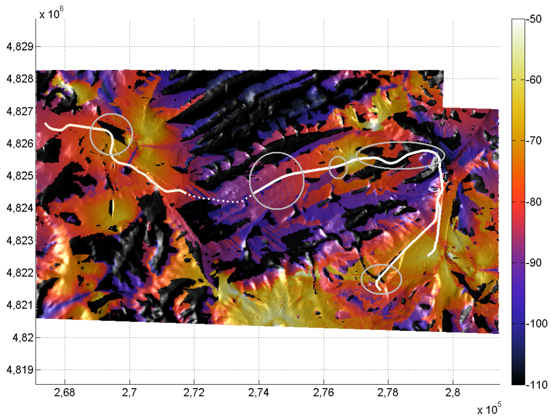
Figura 5.18: Ejemplo en entorno rural (IV). Densidad de potencia para la configuración inicial, [dBW/m 2 ].
