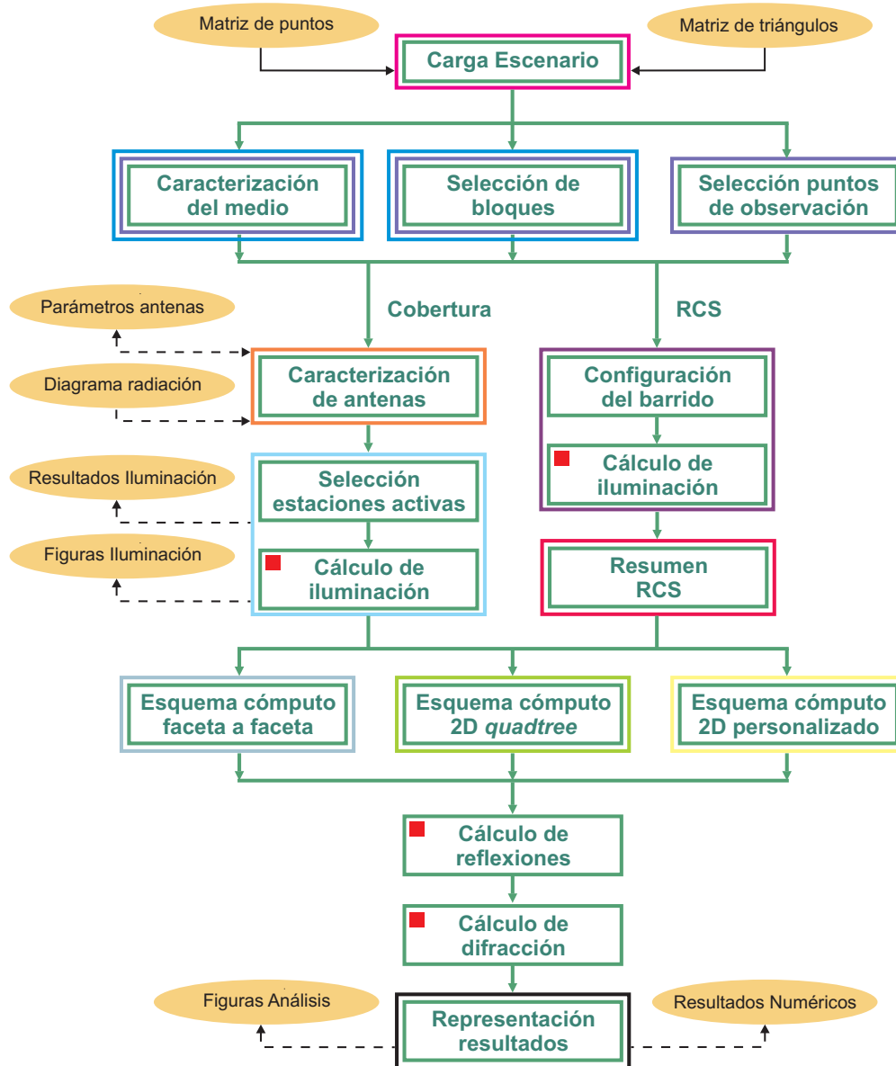
Figura B.1: Diagrama de bloques de la herramienta de cálculo de cobertura.
