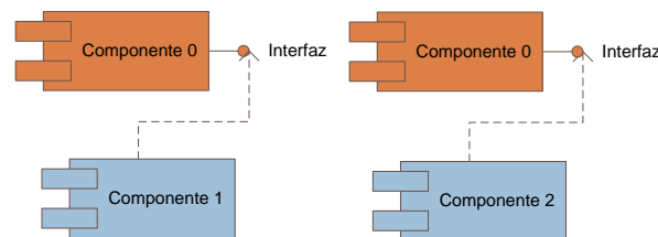
Figura 8.5: Integración con particionado (duplicación de elementos)
