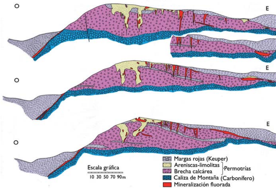
Figura 10. Perfiles característicos del Filón Josefa-Veneros en Veneros Sur (La Collada) (Forster, 1974).
