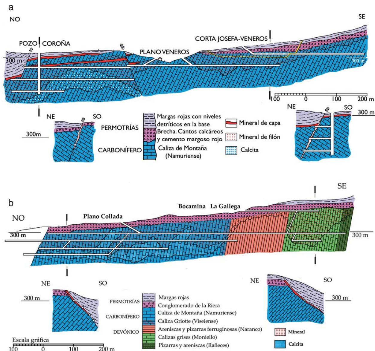
Figura 11. Cortes geológico-mineros –longitudinal y transversales– de los filones Josefa-Veneros (a) y Collada (b), con la disposición de las labores mineras (Tejerina Lobo y Vargas Alonso, 1980).
