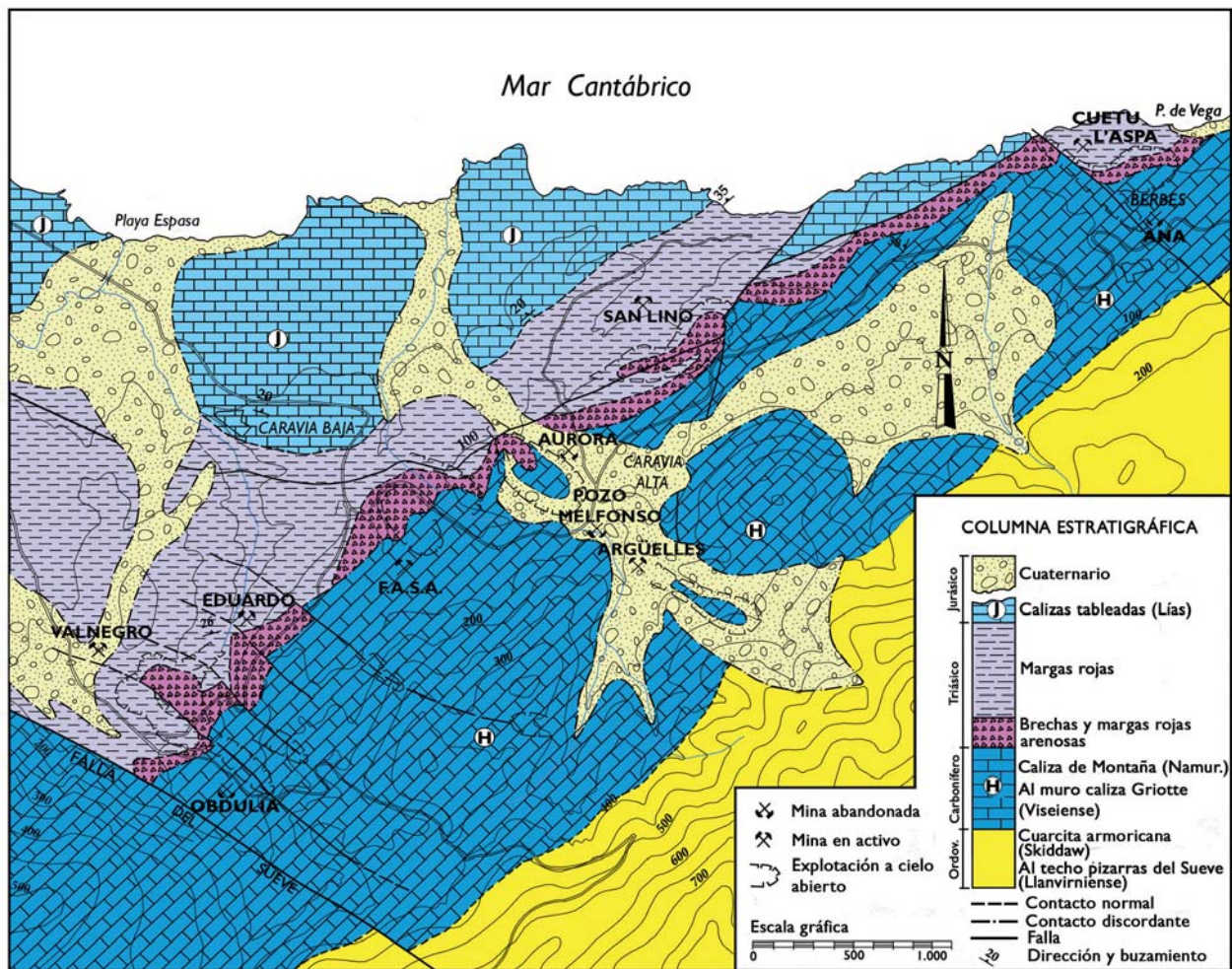
Figura 14. Mapa geológico-minero del Distrito de Caravia-Berbes (Tejerina Lobo y Zorrilla Bringas, 1980).
