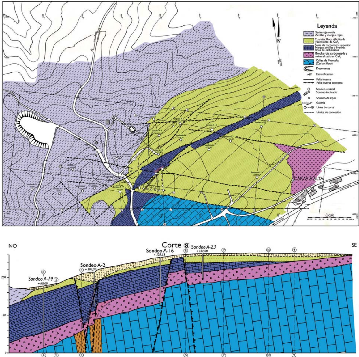
Figura 21. Mapa y corte geológico representativo de la Mina Amalita (Huber, 1976).
