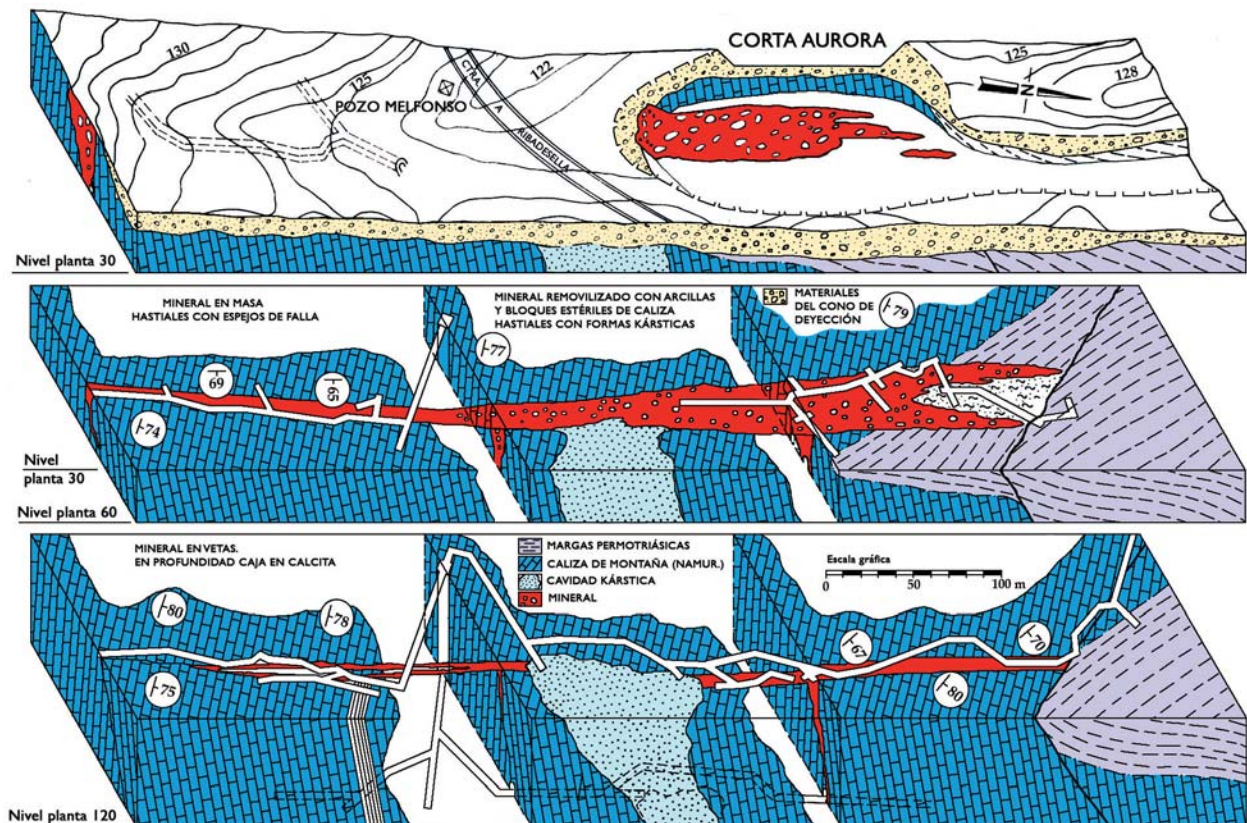
Figura 18. Bloques diagrama representando el trazado del Filón Aurora a distintas cotas en las inmediaciones de la Corta Aurora y del Pozo Melfonso (Tejerina Lobo y Zorrilla Bringas, 1980).
