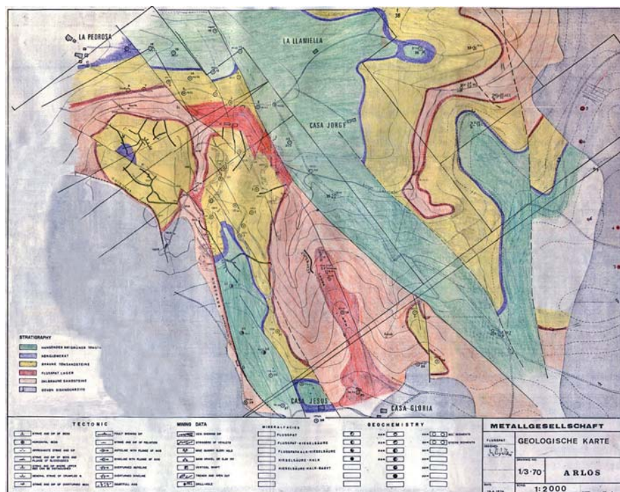
Figura 6. Mapa geológico de la zona de Arlós realizado por la empresa Metallgesellschaft en 1970.
