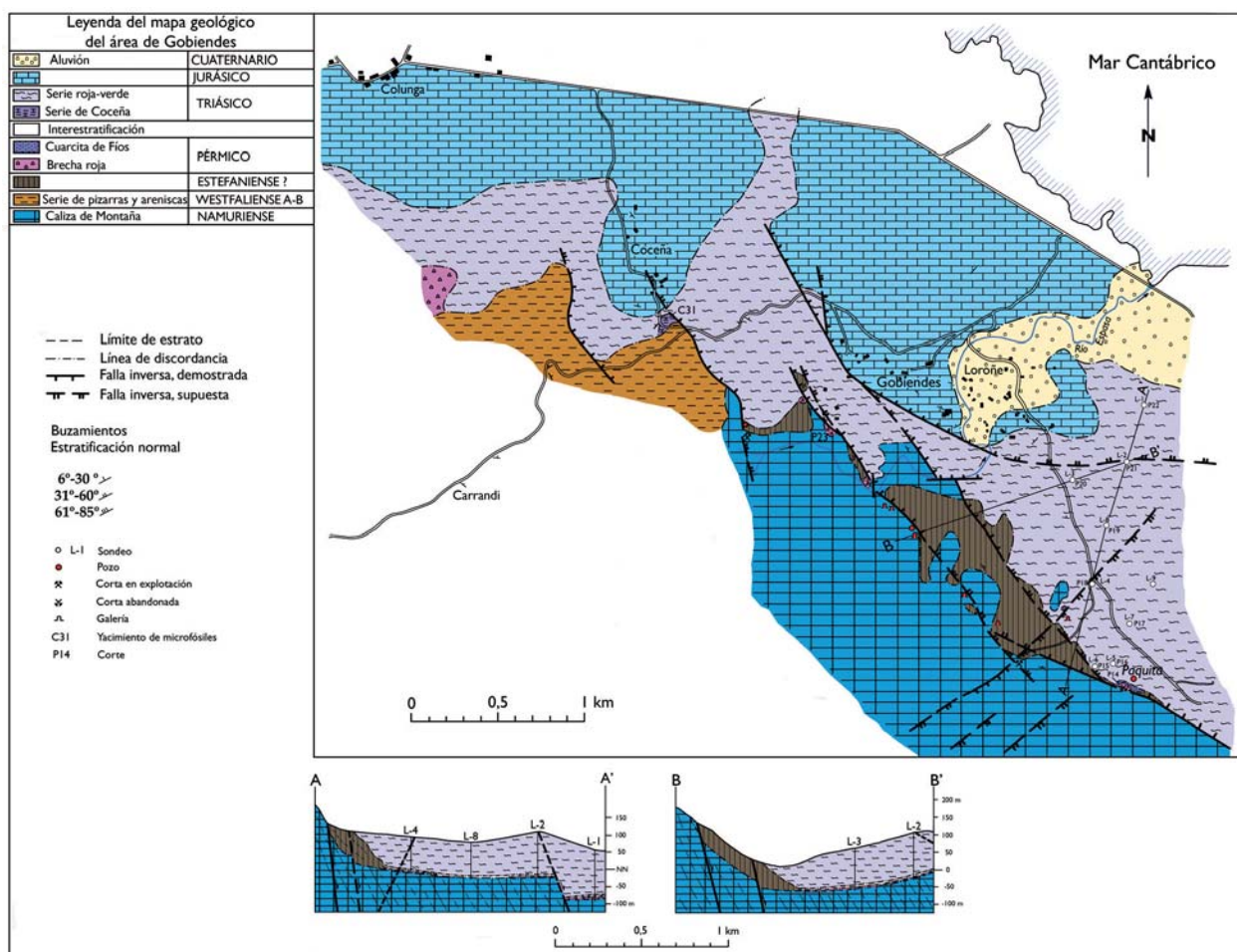
Figura 17. Mapa geol3gico de las inmediaciones de Gobiendes (actualizado de Schäfer, 1974).
