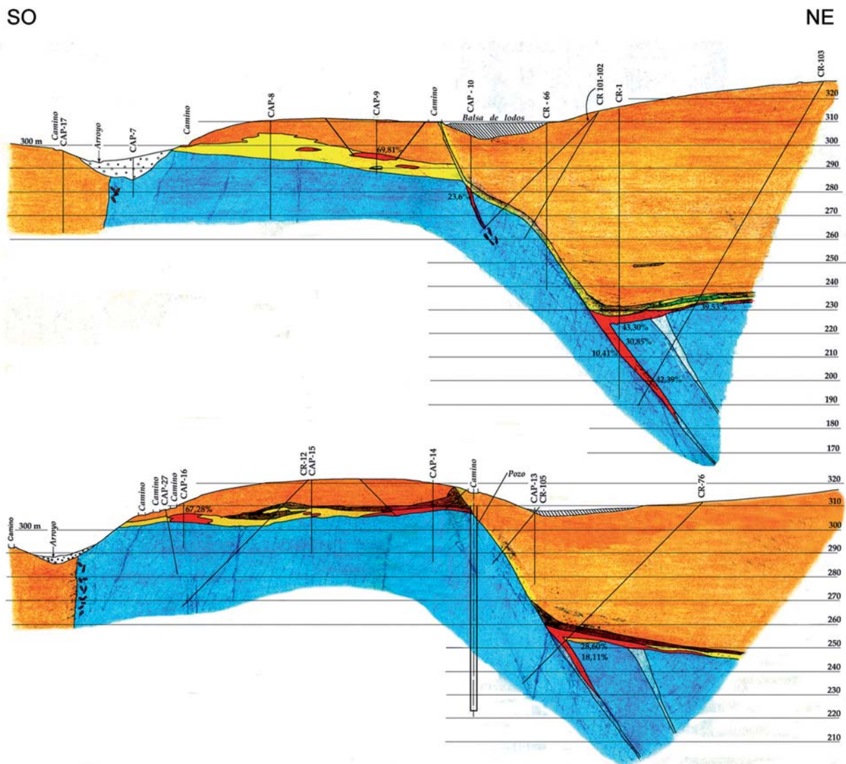
Figura 3. Distribución de la mineralización (en rojo) en el Filón Josefa-Veneros y estratoligada en la zona de Coruña. (Según informes internos de Fluoruros, S. A. del año 1974).
