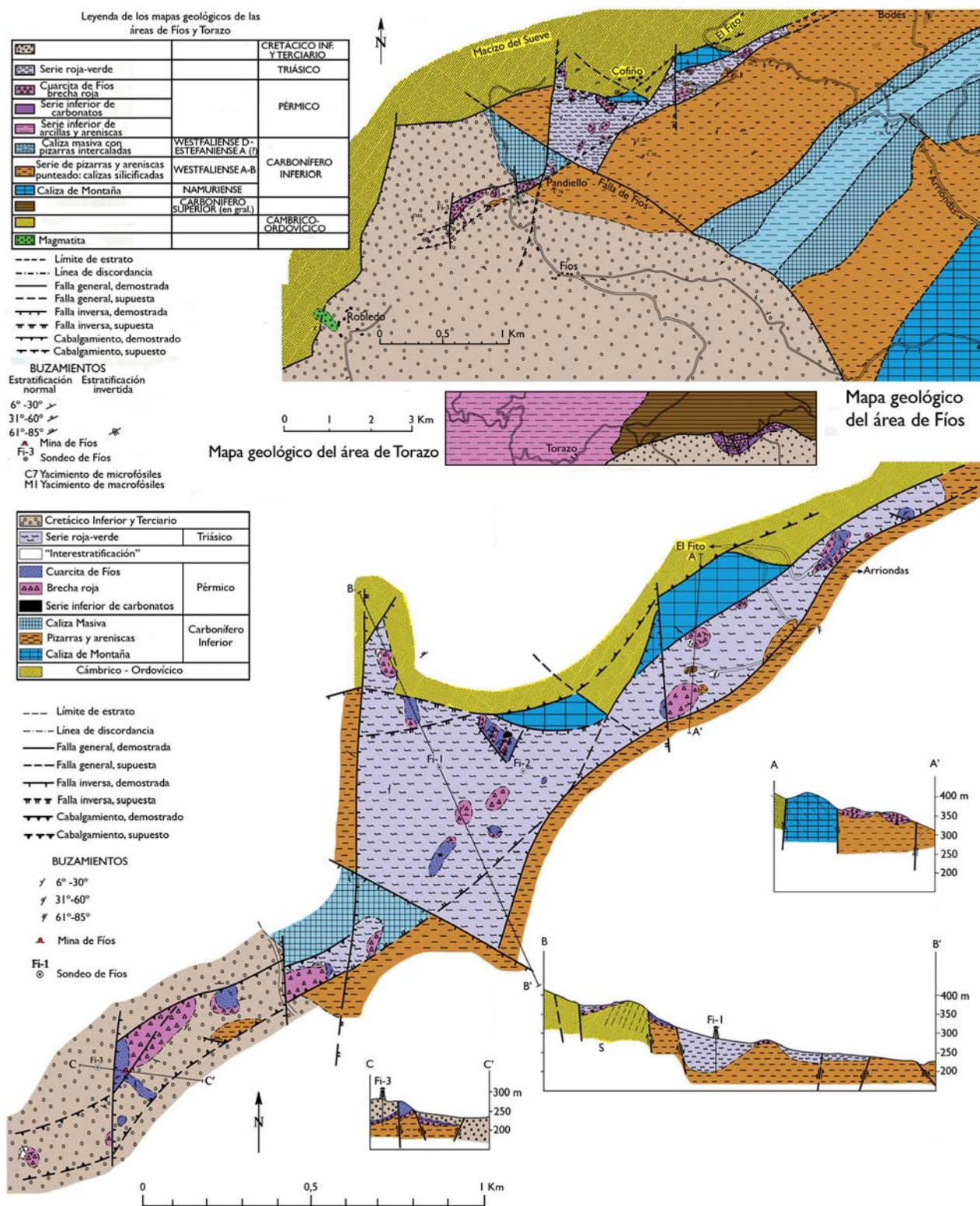
Figura 22. Mapas geológicos de los alrededores de Fíos, a diferentes escalas, y de Torazo (Schäfer, 1974).
