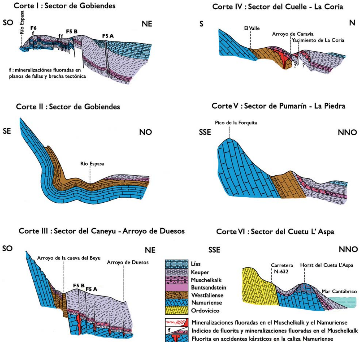
Figura 15. Cortes geológicos de Caravia-Berbes. Véase situación en figura 12 (Jullien, 1974).
