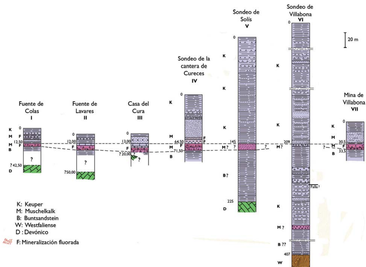
Figura 4. Columnas estratigráficas representativas del Distrito de Villabona-Arlós (Jullien, 1974).
