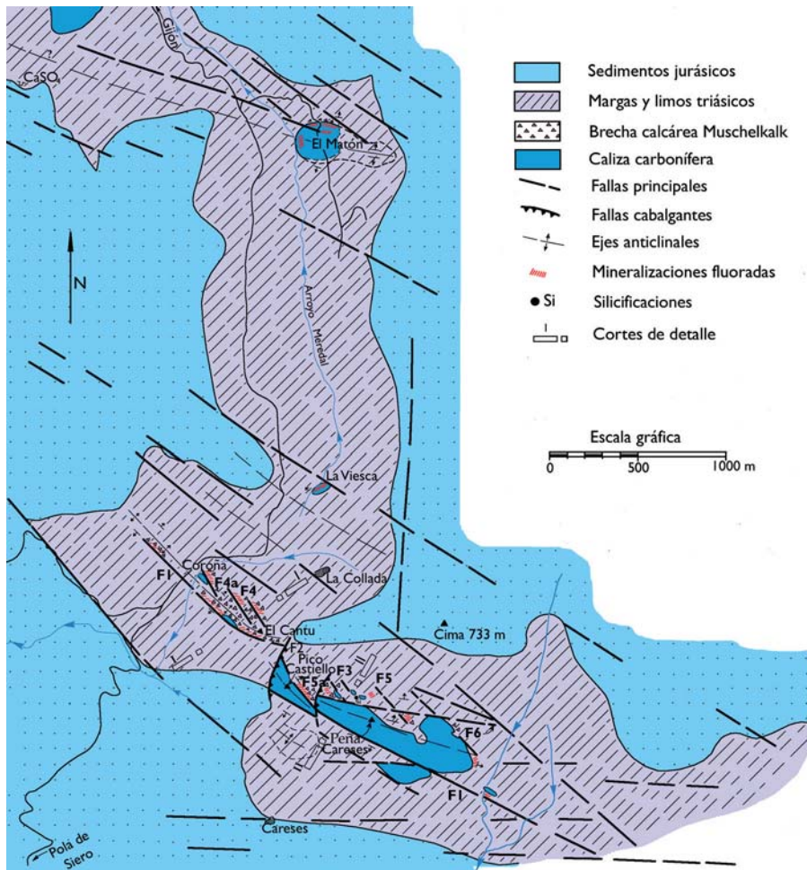
Figura 7. Esquema geológico del Distrito de La Collada (Jullien, 1974).
