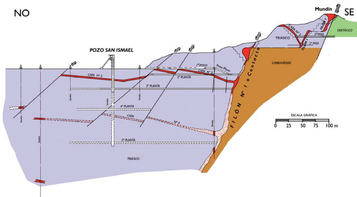
Figura 2. Corte geológico-minero mostrando la disposición de las capas y filones en el yacimiento de Villabona (documentación inédita de la empresa Minas de Villabona). Nota: en rojo mineralización de fluorita.
