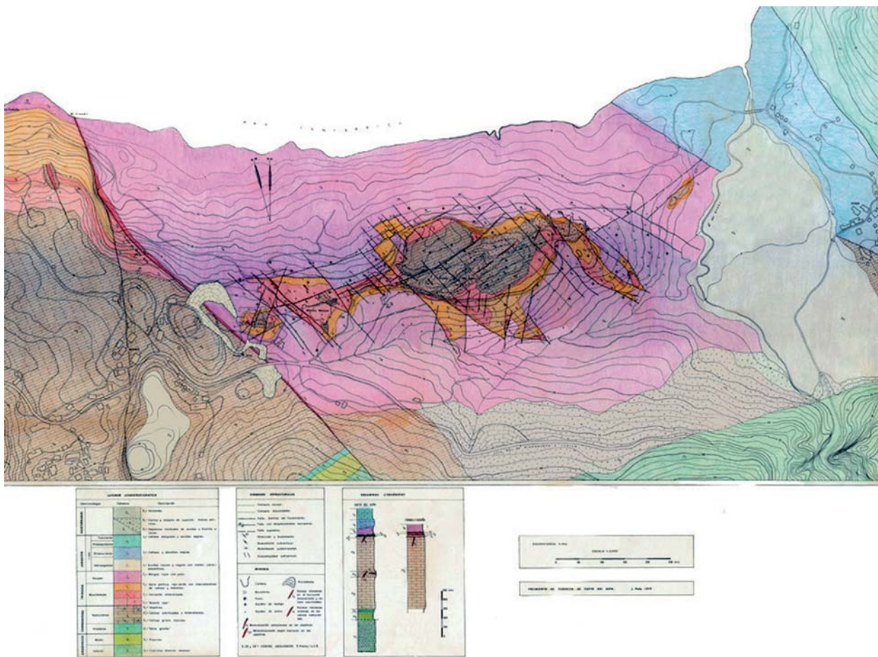
Figura 19. Mapa geológico de Cuetu l'Aspa. Nótese la gran densidad de fracturas (Peña Barbero, 1981).
