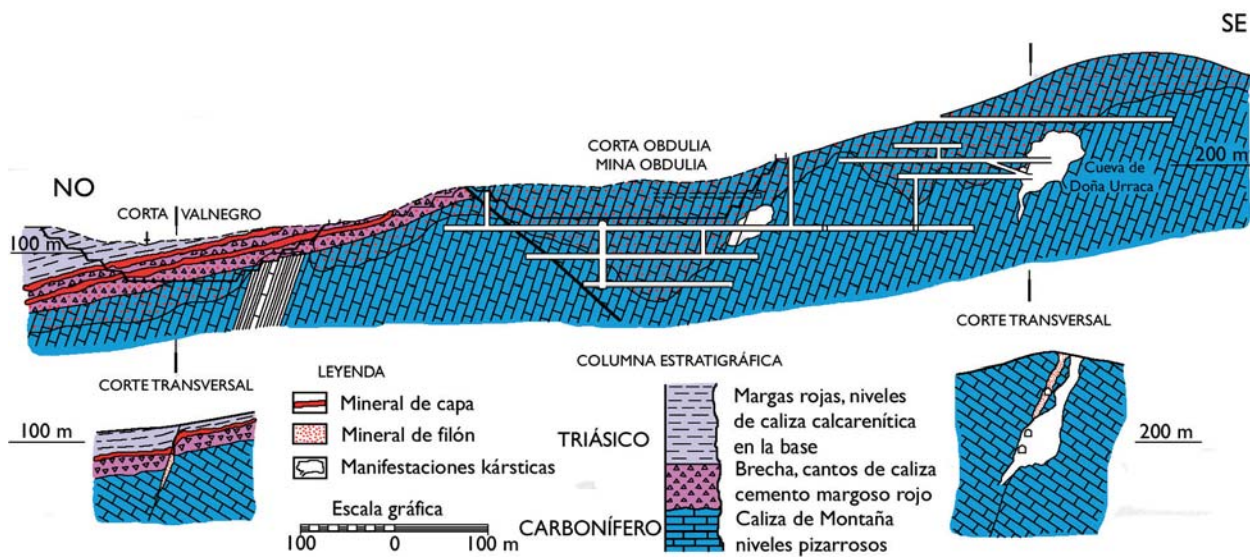
Figura 16. Cortes longitudinales y transversales en el entorno de Mina Obdulia-Corta Valnegro (Tejerina Lobo y Zorrilla Bringas, 1980). Nota: La parte superficial (punteada en rojo) corresponde al Filón Obdulia.
