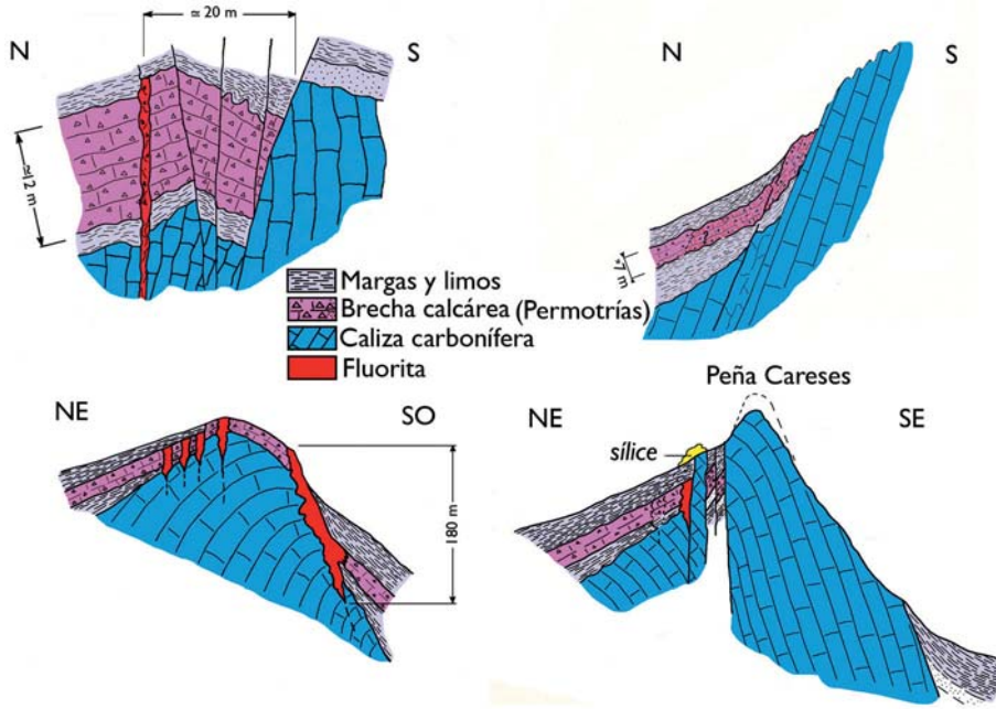
Figura 9. Cortes geológicos esquemáticos en el Distrito de La Collada poniendo de manifiesto las particularidades del contacto Permotriás-Carbonífero (Jullien, 1974).
