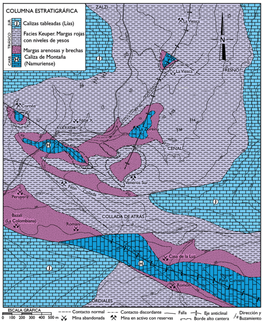
Figura 8. Esquema geológico del Distrito de La Collada (Tejerina Lobo y Vargas Alonso, 1980).
