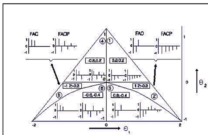
Gráfica 1: Regiones de estacionariedad para los procesos AR(2). (Según Stralkowsky, Wu y Devor, 1970).
