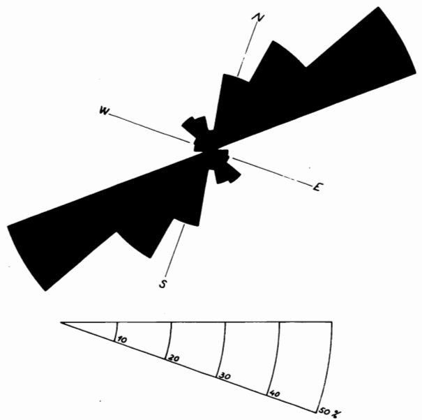
Fig. 3. Diagrama de rumbos de fracturas en el valle de Tánago (muestra: 84 fracturas).
