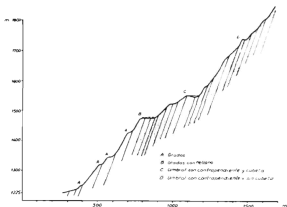
Fig. 8. Perfil de las formas de excavación principales en el fondo del valle glaciar del Tánago (tengase en cuenta la exageración de la escala vertical y el consiguiente enderezamiento de las capas sedimentarias).
