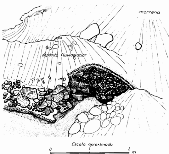
Fig. 16. Corte en las canteras del Hoyo del Tejo: depósitos fluvio-glaciares deformados bajo la morrena depositada por el lóbulo glaciario difluente de Valdiezmo.
