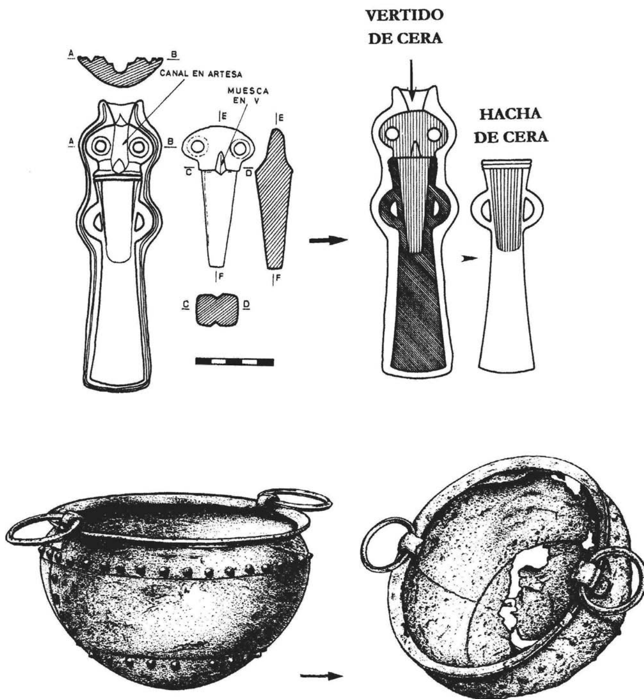
Figura 9. Molde de Los Oscos (según M. A de Blas) y caldero de Cabárceno antes y después de su restauración (según Fernández, Guerra, 2003).
